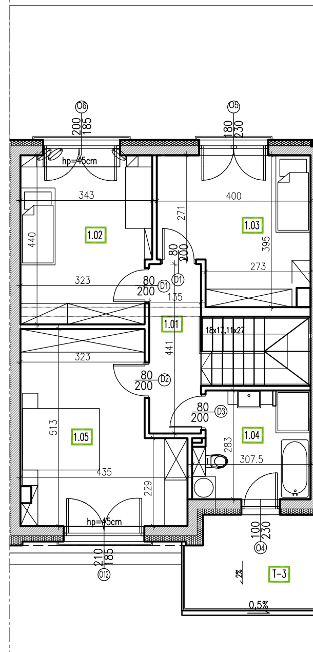
ZESTAWIENIE POWIERZCHNI PIĘTRA
