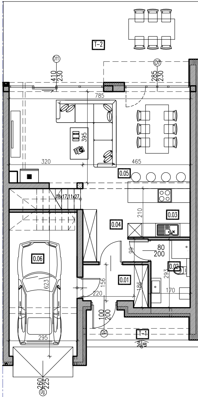
ZESTAWIENIE POWIERZCHNI PARTERU
